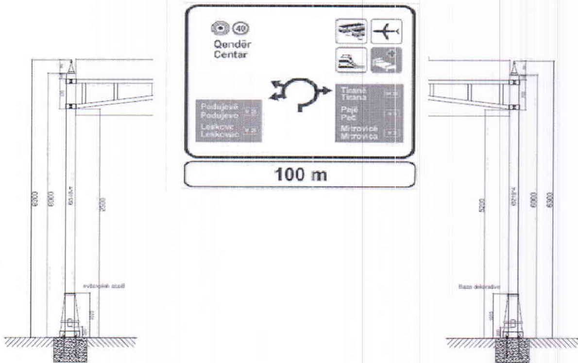
Figura 5. Dimensionet e semaforëve portal
